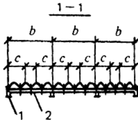
Черт. 14. Схема плиты из гофрированного листа с продольными и поперечными ребрами 1 - продольные ребра; 2- поперечные ребра
