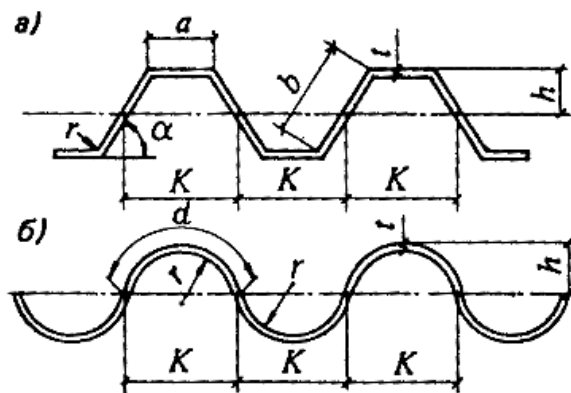
Черт. 13. Геометрические параметры для гофра
