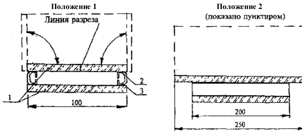
Рисунок 8 — Испытание герметика первого герметизирующего слоя
