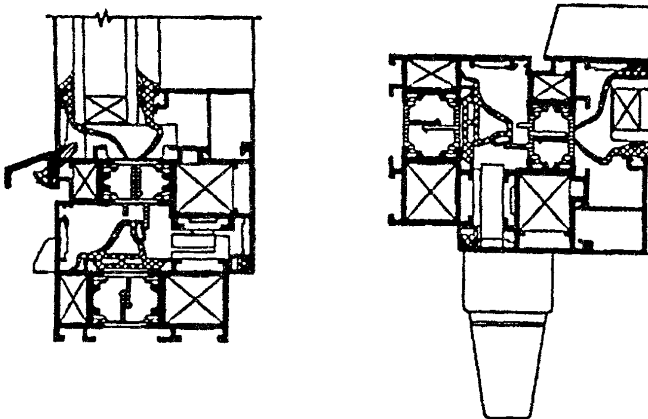
Рисунок 3 — Вариант конструктивного решения узлов притвора оконного блока с поворотно-откидным открыванием внутрь по
